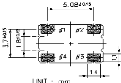
UNIT : mm
